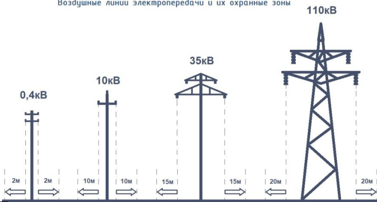
Воздушные линии электропередачи и их охранные зоны
